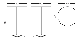
Ø60 x H95 cm
